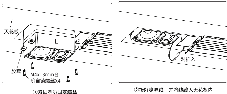
① 紧固喇叭固定螺丝
