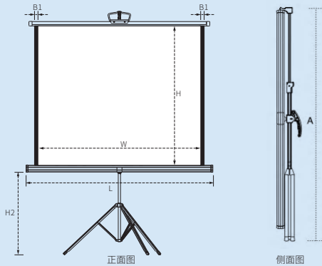
正面图
